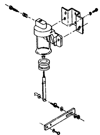
OUD-160 Air Dashpot Assembly
