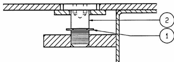
EZ-LIFT™ - Hold-Down Bolt
