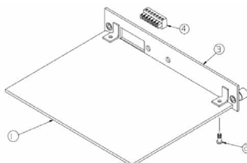
IDNet PCB
