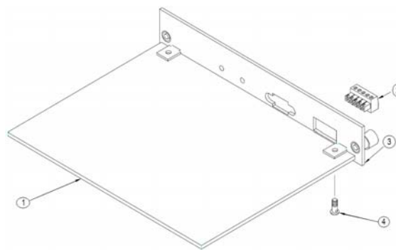
Modbus Plus PCB Assembly
