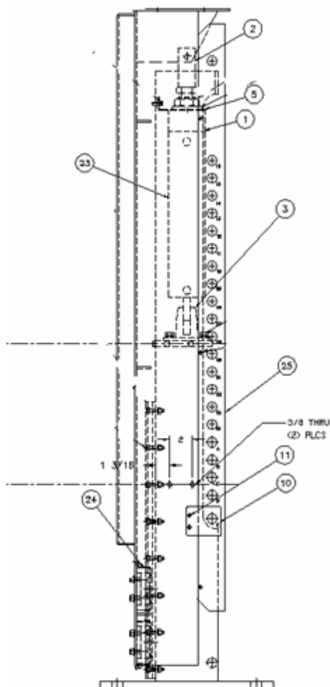
9127 - Surface Top Fill RAM Assembly
