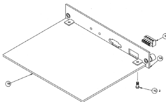
MODBUS Plus PCB
