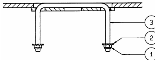
EZ-LIFT™ - Lift Handle
