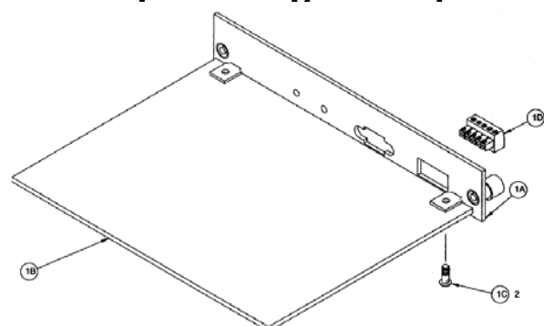
PROFIBUS Option
