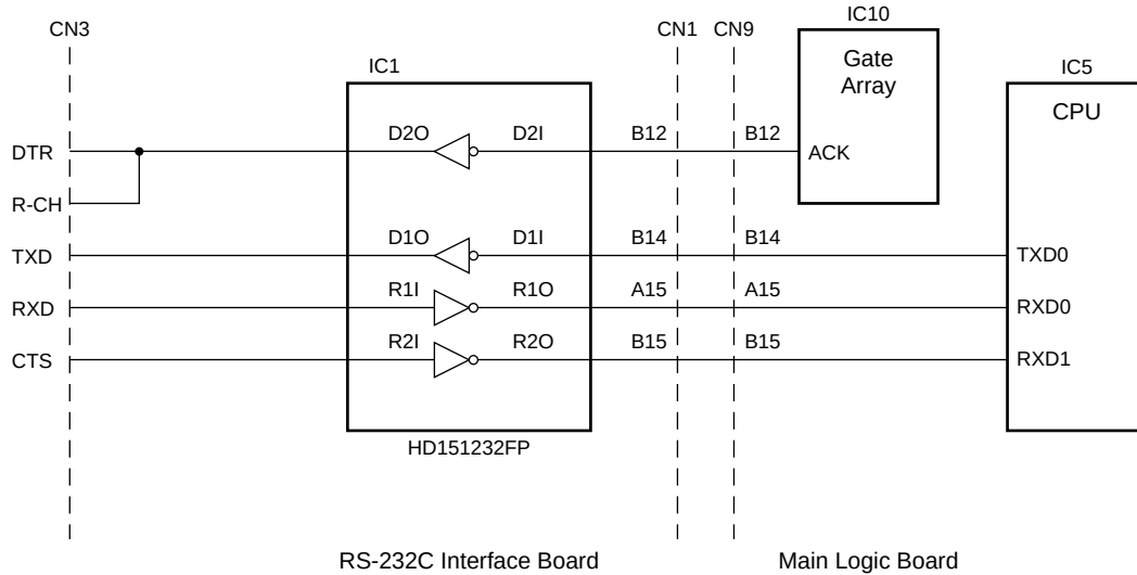
Fig. 2-2 RS-232C Interface
