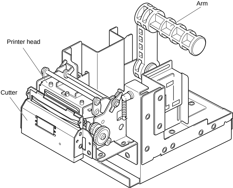
Fig. 1-2-a Internal Configuration (TUP452)
