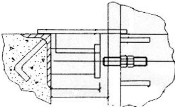
Bumper bolt / Boulons de butée
