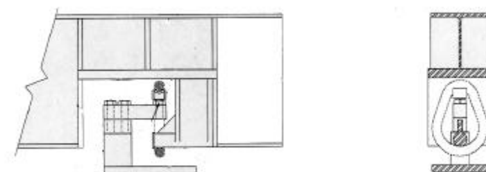
Load cell mounting / Montage de la cellule de pesage
