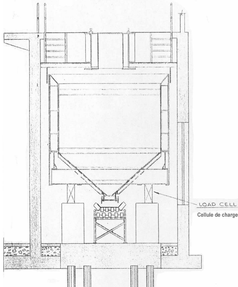
Hopper scale/ Trémie de pesage
